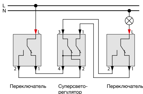
Имеющаяся схема включения и выключения суперсветорегулятора
