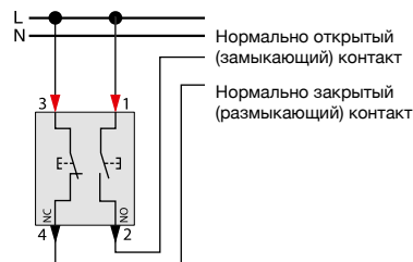
2-кнопочный выключатель, 1 замыкающий контакт, 1 размыка- ющий контакт MTN3153-0000
