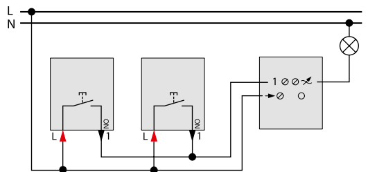
Схема светорегуляции с промежуточным и кнопочным выключателями
